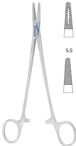
MAYO HEGAR NEEDLE HOLDER
